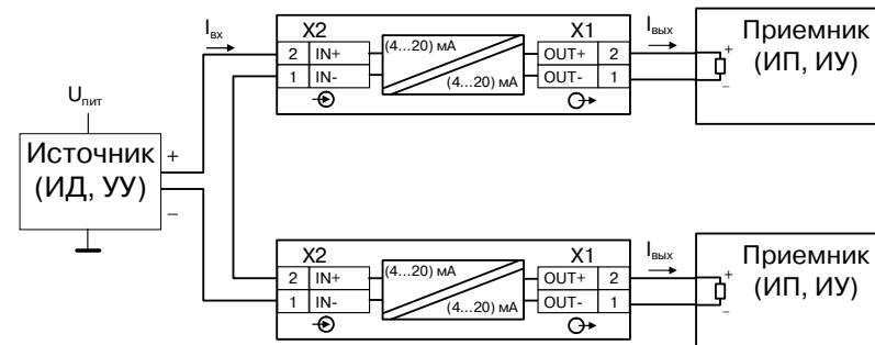
Рисунок 5.7 – Разделение сигнала от одного датчика на два гальванически изолированных при помощи двух НПСИ-200-ГРТП1
