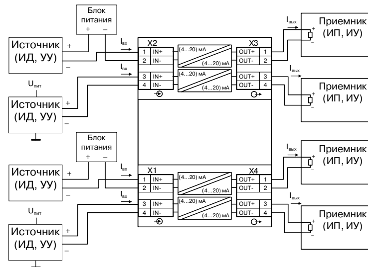
Рисунок 5.6 – Типовое подключение НПСИ-200-ГРТП4
