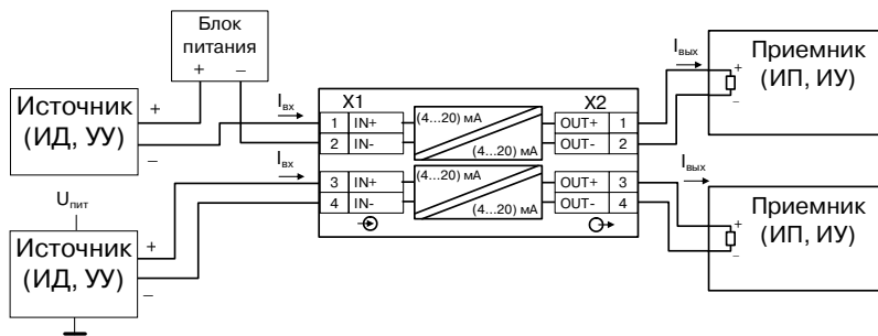
Рисунок 5.5 – Типовое подключение НПСИ-200-ГРТП2
