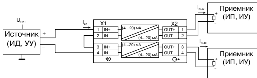
Рисунок 5.8 – Разделение сигнала от одного датчика на два гальванически изолированных при помощи НПСИ-200-ГРТП2
