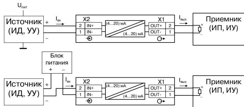
Рисунок 5.4 – Типовые подключения НПСИ-200-ГРТП1
