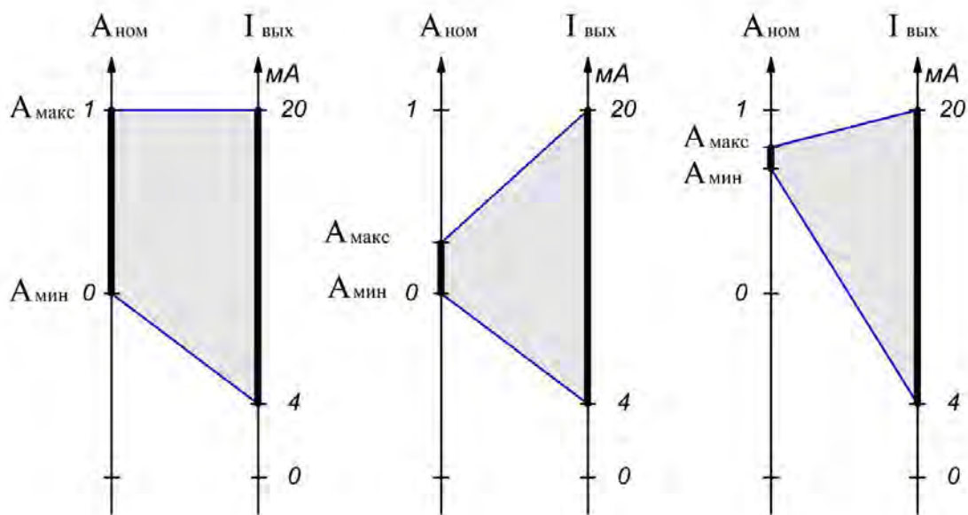
в) – (4...20) МА
