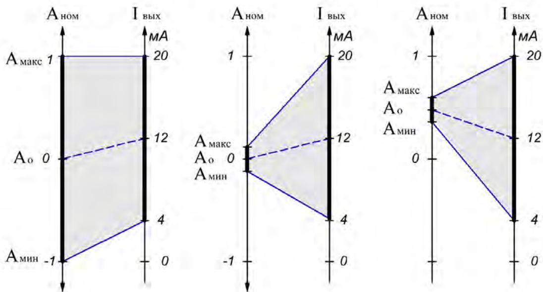
г) – (4...12...20) МА
