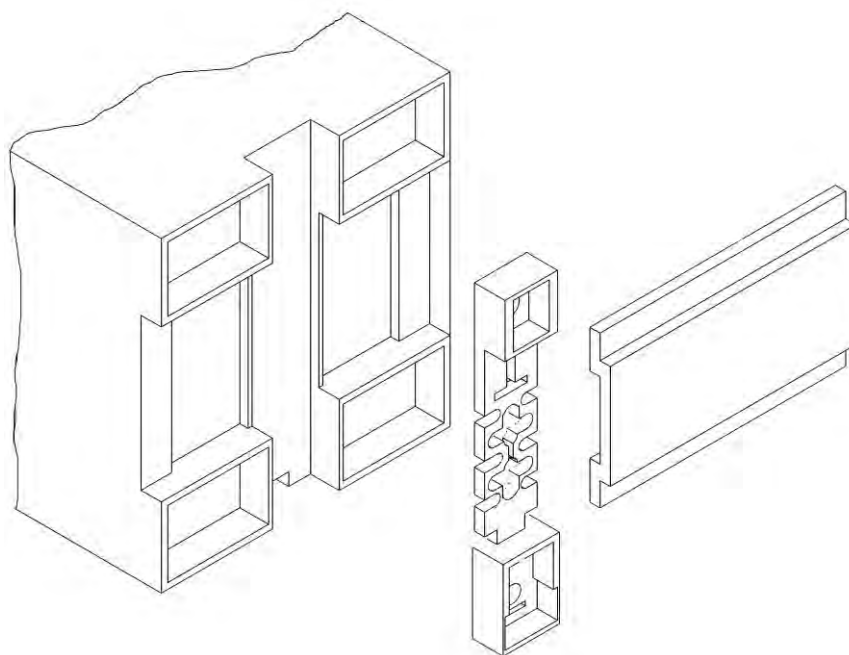
Рисунок 6 – Крепление преобразователя на DIN-рейку
