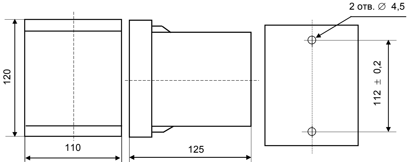
Рисунок Б.1 – Габаритные и установочные размеры ИП ЭП8554/3, ЭП8554/4, ЭП8555/3-ЭП8555/5, ЭП8555/7
