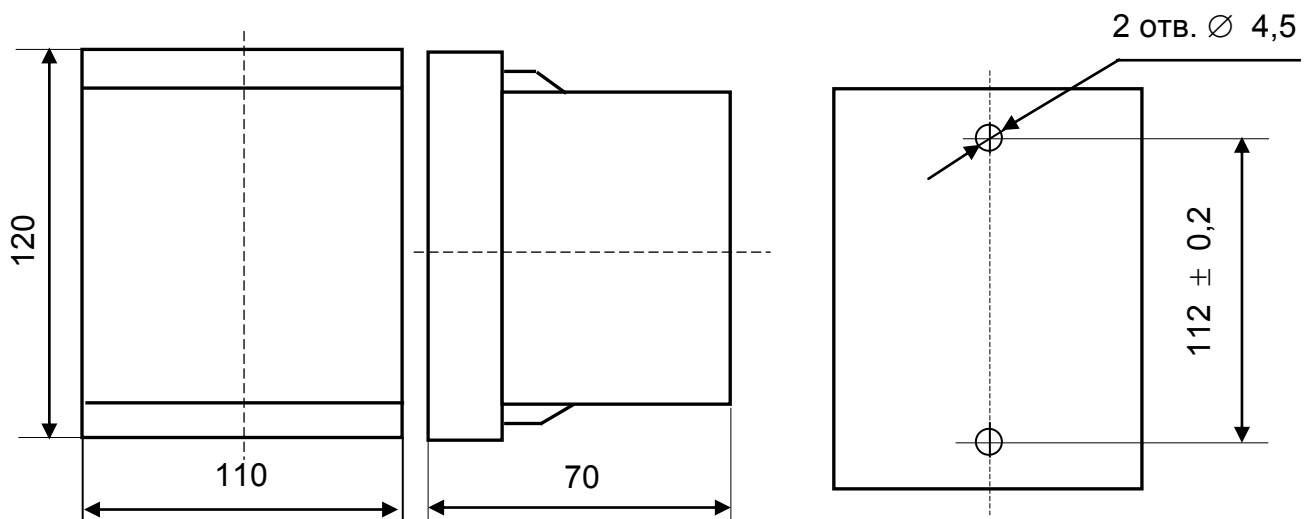
Рисунок Б.2 – Габаритные и установочные размеры ИП ЭП8554/1, ЭП8554/2, ЭП8554/5, ЭП8554/6, ЭП8555/1, ЭП8555/2, ЭП8555/6, ЭП8555/8, ЭП8555/9
