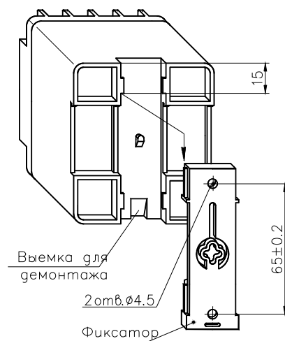
Рисунок Б.2 Вариант крепления на панель
