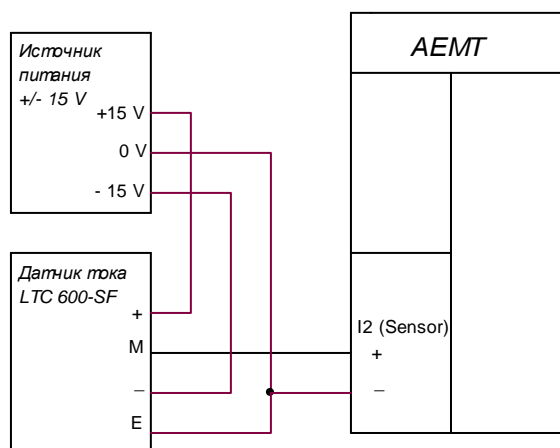
Рисунок Д.2 Пример подключения датчика тока к измерительной цепи преобразователя
