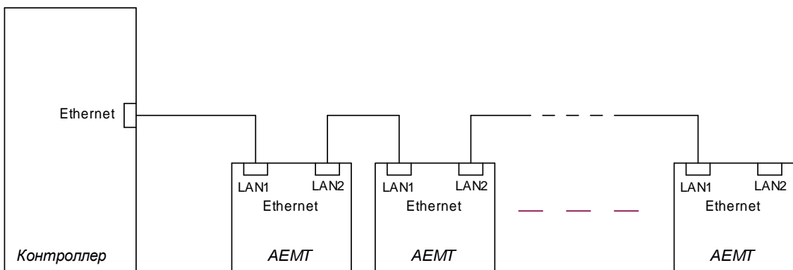
Рисунок Д.5 Подключение преобразователей к интерфейсу Ethernet контроллера телемеханического комплекса
