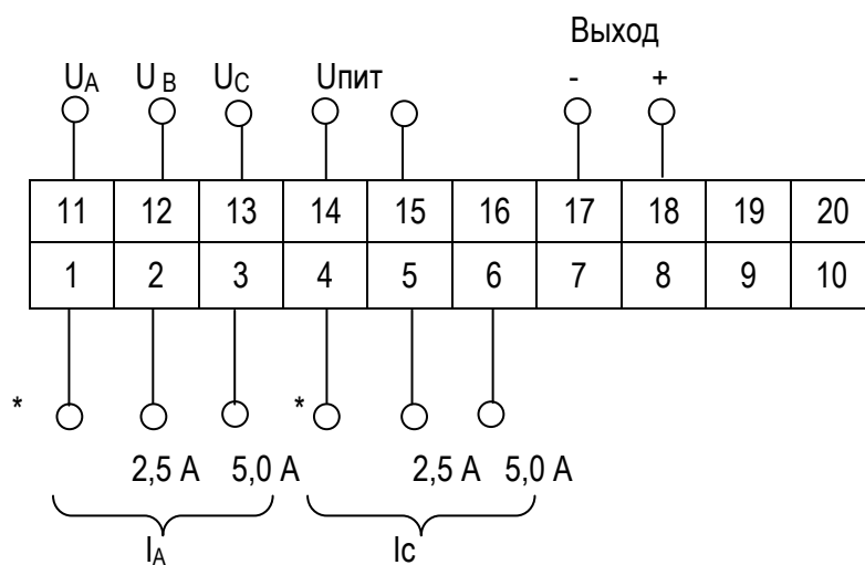
Рисунок А.2 – Схема подключения ИП E 860/2ЭС, E 860/4ЭС, E 860/5ЭС, E 860/7ЭС, E 860/10ЭС
