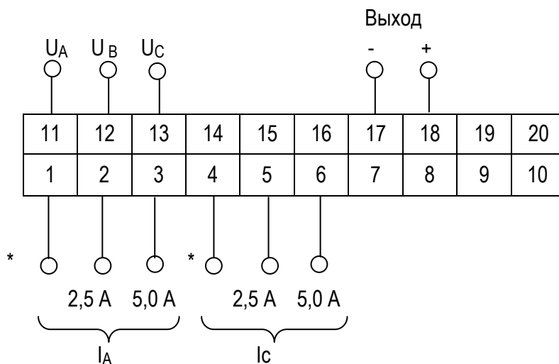
Рисунок А.3 – Схема подключения ИП E 860/1ЭС, E 860/3ЭС, E 860/6ЭС, E 860/8ЭС, E 860/9ЭС
