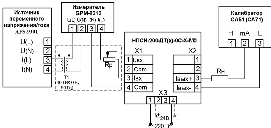
Рисунок А.6.3.2 – Подключение преобразователей НПСИ-200-ДТ для проведения поверки преобразования переменного тока в ток от 4 до 20 мА
