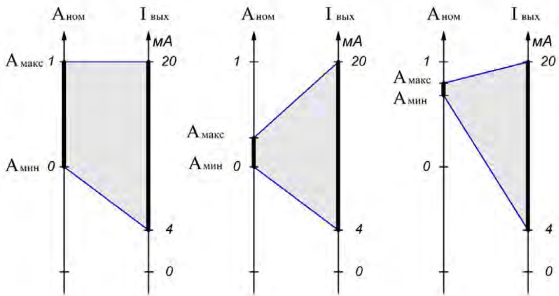
в) – (4...20) МА
