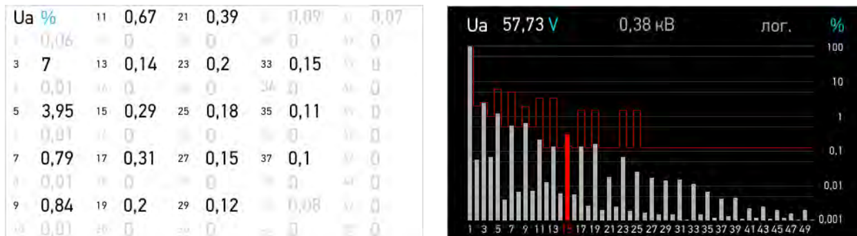
Рисунок 5.21. «ПКЭ» -> «Гармоники».
