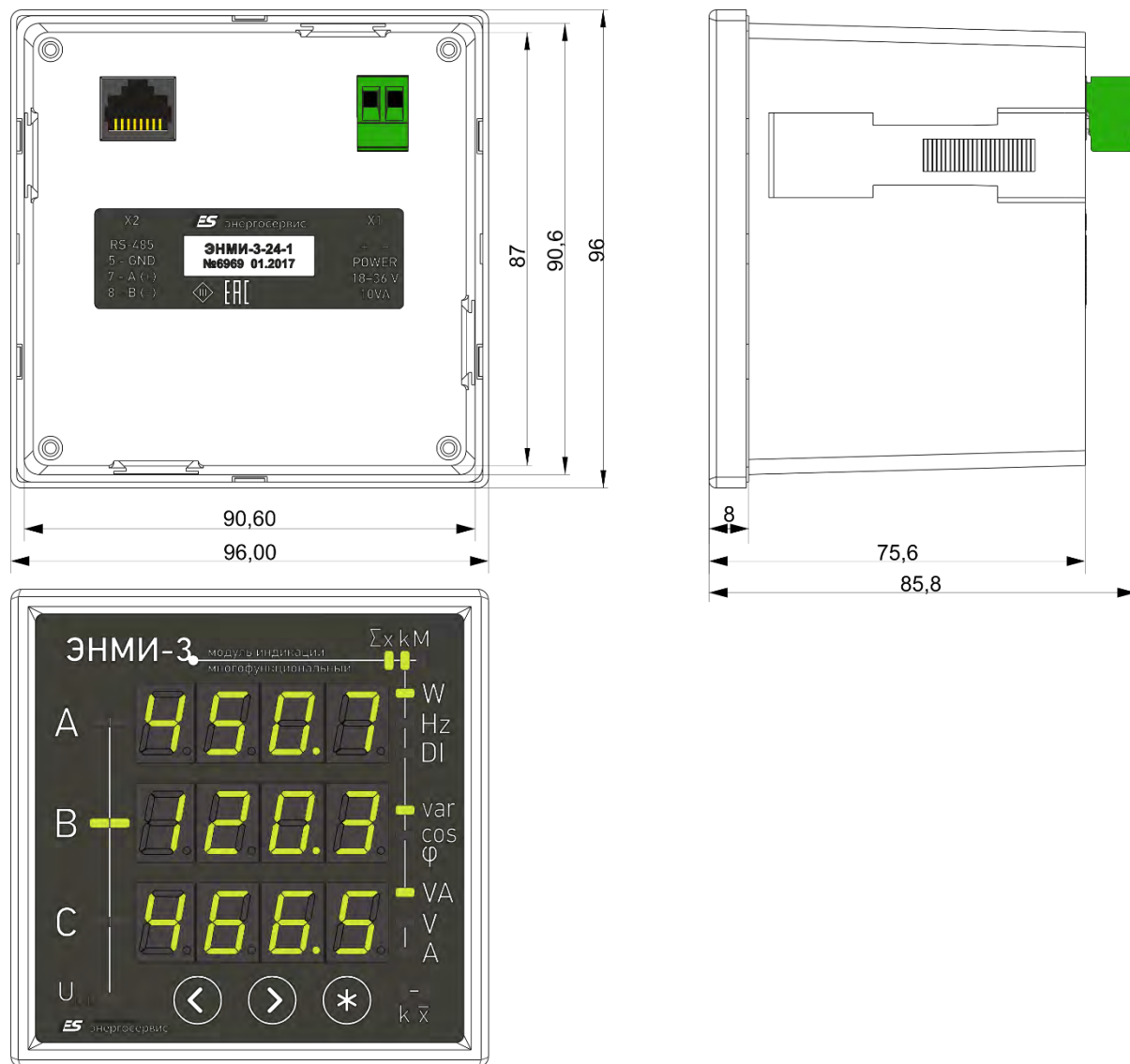
Рисунок 2.1. Габаритные размеры модификации ЭНМИ-Х-24-1.
