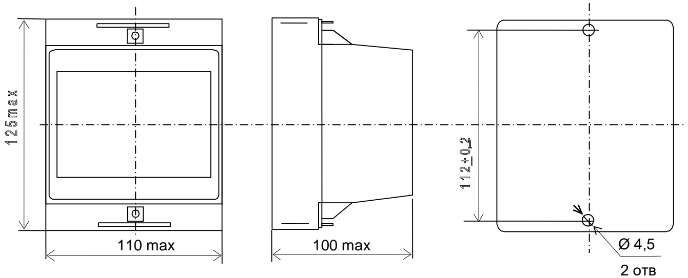
Рисунок А.1 – Габаритные и установочные размеры ИП
