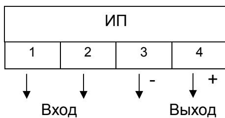
Рисунок Б.1 – Схема электрическая подключения
