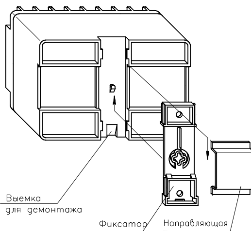
Рисунок Б.1 Вариант крепления на направляющую
