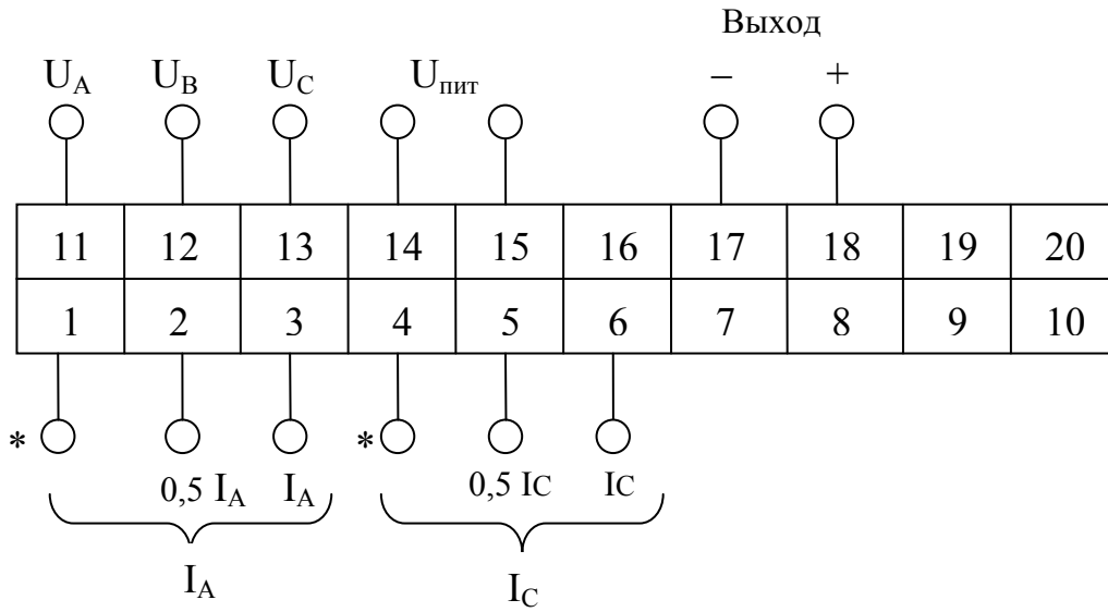
Рисунок А.5 – Схема подключения ИП E848M/6, E848M/7, E848M/9, E848M/11, E848M/12
