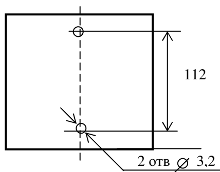
Рисунок А.1 – Габаритные размеры ИП
